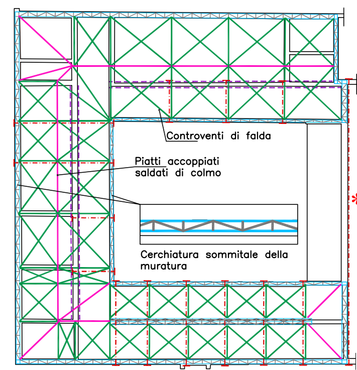
VARIANTE - PIANTA CARPENTERIA METALLICA
